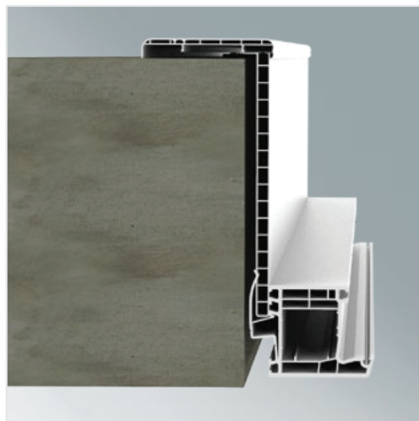
2 Sistema a giunzione angolare retto con Profilo scatolato su intradosso interno
